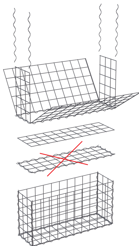
PŘÍKLAD MONTÁŽE GABIONOVÝCH KOŠŮ NA SEBE
